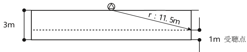
〔側面図〕
