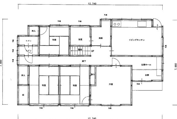
1階平面図
