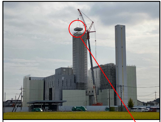
② 3号炉焼却棟 煙突外筒撤去
