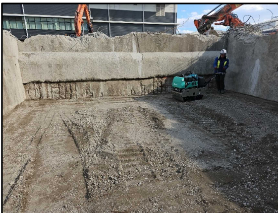
① 3号炉焼却棟 ごみピット埋戻し
