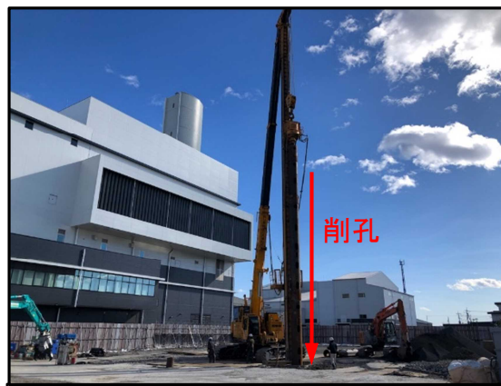
④ 粗大ごみ処理施設 杭抜き (削孔)
