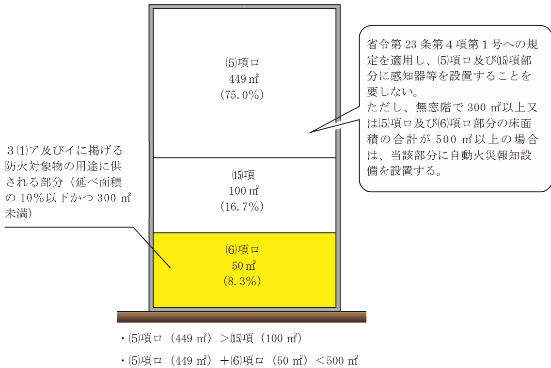
(小規模特定用途複合防火対象物 (16項イ))
