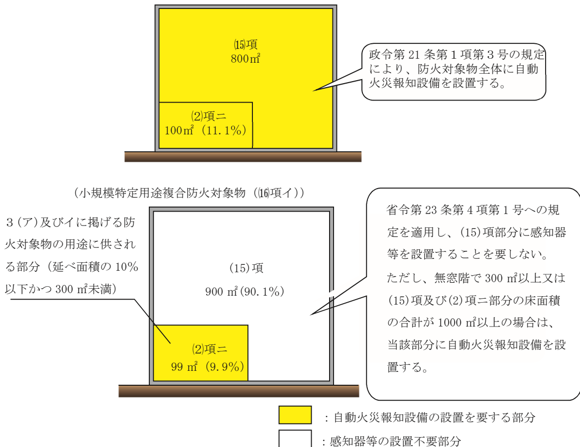
例1（複合用途防火対象物（16項イ））
