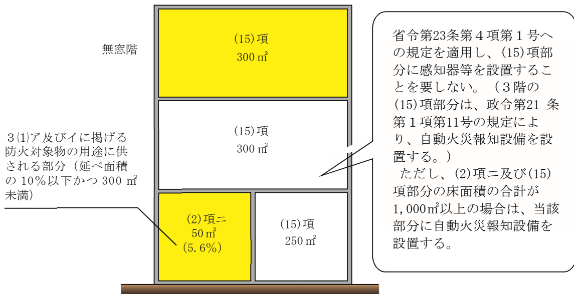
(小規模特定用途複合防火対象物 (16項イ))
