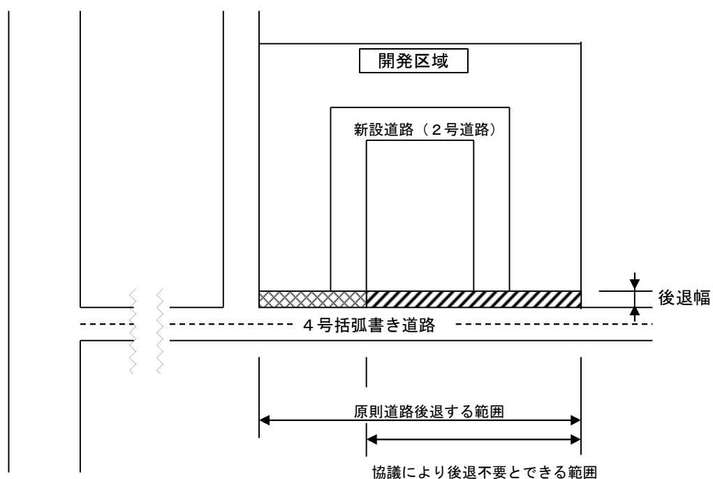
図－１１－２ 「道路後退する範囲」の扱い
