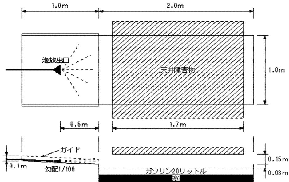
第21-5図 水平放出方式試験装置
