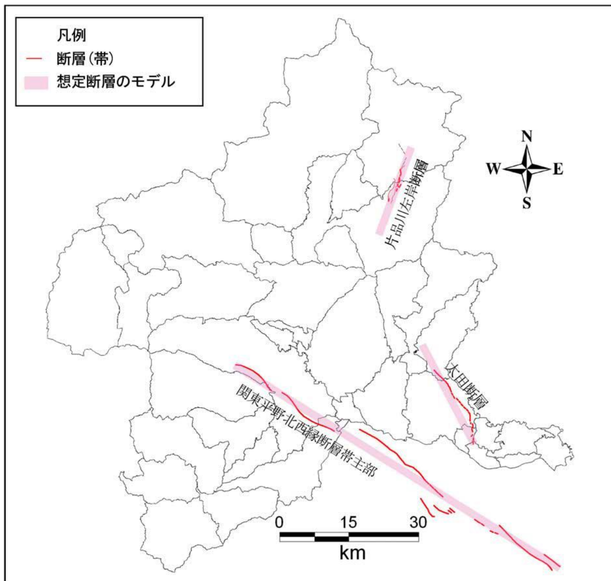
<想定地震の震源断層位置図>
