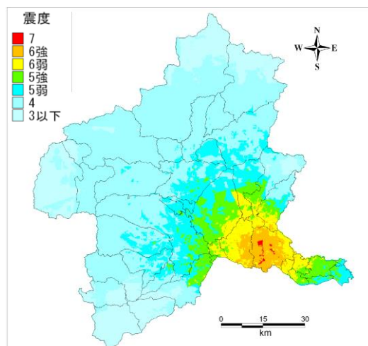
＜太田断層による地震(M7.1)の場合の地表震度分布図＞
