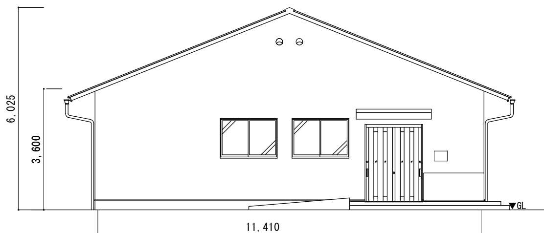
東立面図
