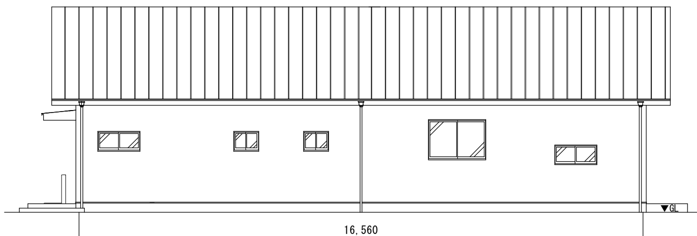
北立面図
