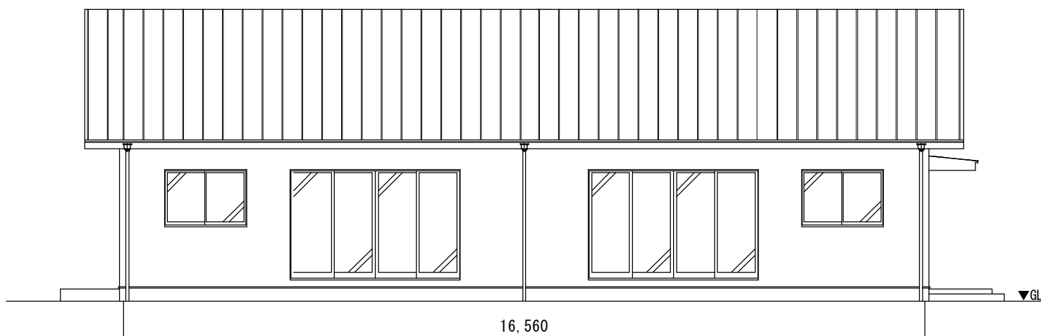
南立面图
