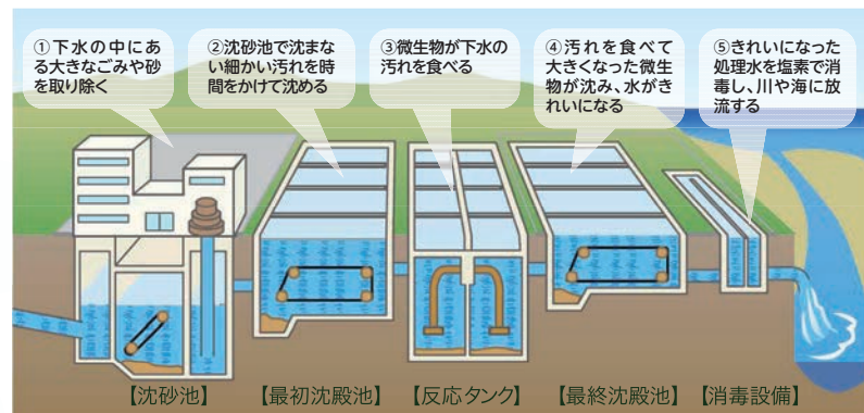
▲下水処理場
